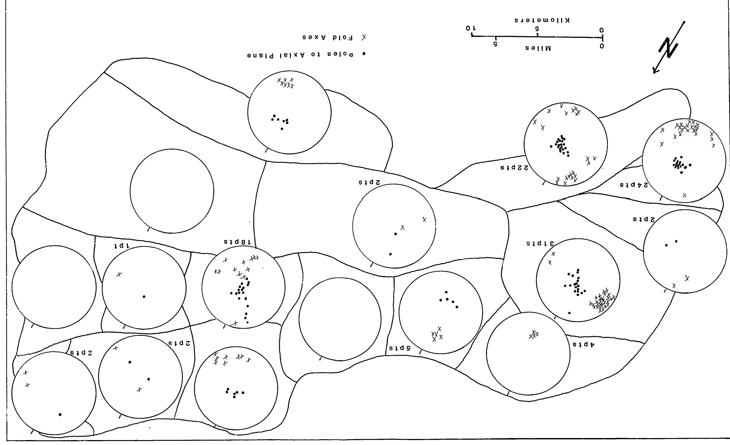
Plate 1e Stereographic plots, F1 folds
