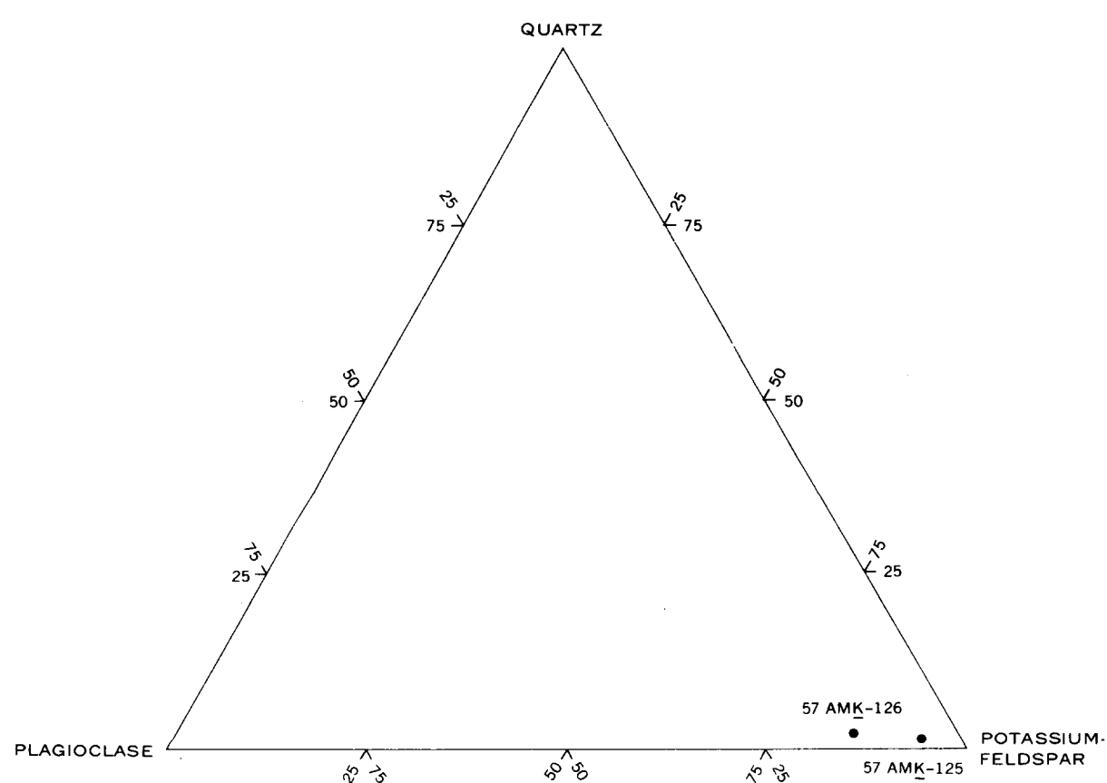
E. SYENITE
