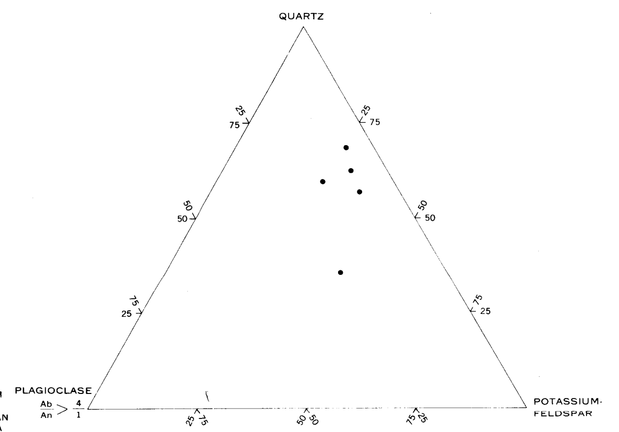
G. APLITE
